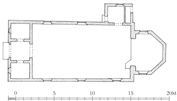
Fig. 7. Grundplan. 1:300. Målt og tegnet af Pia K. Lindholt 2023. Signaturforklaring s. 9. – Plan. Key on p. 17.
