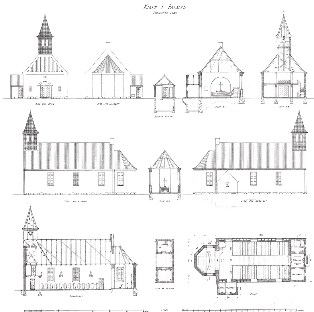
Fig. 8a-k. Tegninger til kirkens opførelse. 1:400. a. Sydvestfacade. b. Nordøstfacade. c. Tværsnit gennem sakristi set mod sydøst. d. Tværsnit gennem skib set mod nordøst. e. Tværsnit gennem kirkens sydvestende set mod sydvest. f. Sydøstfacade. g. Tværsnit gennem kor set mod nordøst. h. Nordvestfacade. i. Længdesnit set mod nordvest. j. Plan af pulpitur. k. Grundplan. Tegnet af Thorvald Nygaard 1931. I kirkens arkiv. — Scale drawings for the construction of the church, 1931. 1:300. a. Southwest facade. b. Northeast facade. c. Cross-section through the sacristy looking southeast. d. Cross-section through the nave looking northeast. e. Cross-section through the southwestern end of the church looking southwest. f. Southeast facade. g. Cross-section through the chancel looking northeast. h. Northwest facade. i. Longitudinal section looking northwest. j. Plan of gallery. k. Plan.
